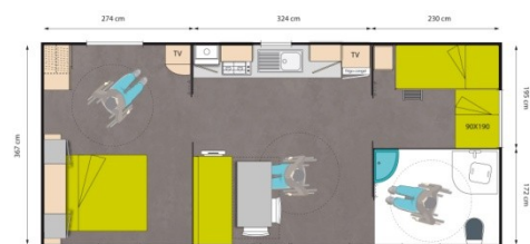
Superficie 28m 2 , année 2012 Plan1/114 ème Les photos et plan ne sont pas contractuels
